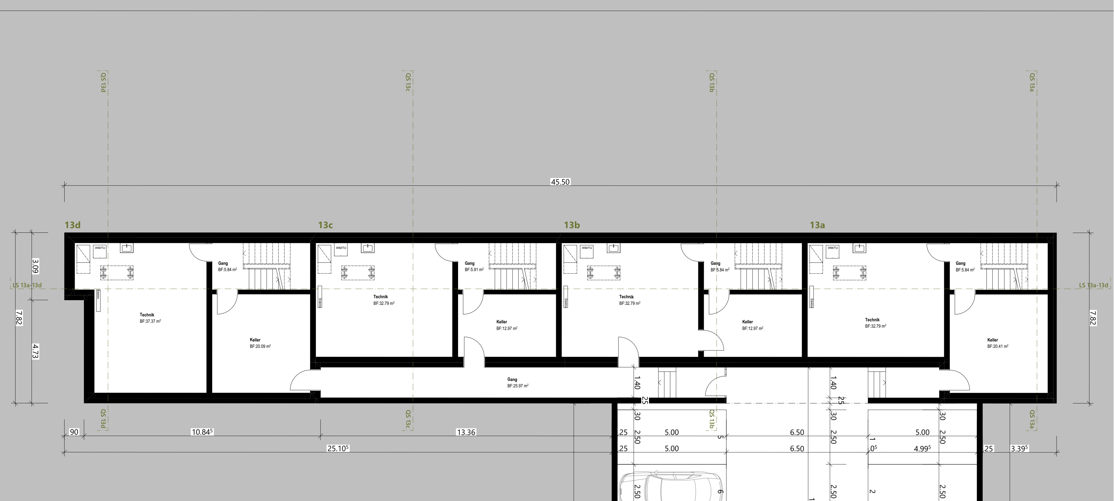
Haus 13a, 13b, 13c und 13d - Untergeschoss
