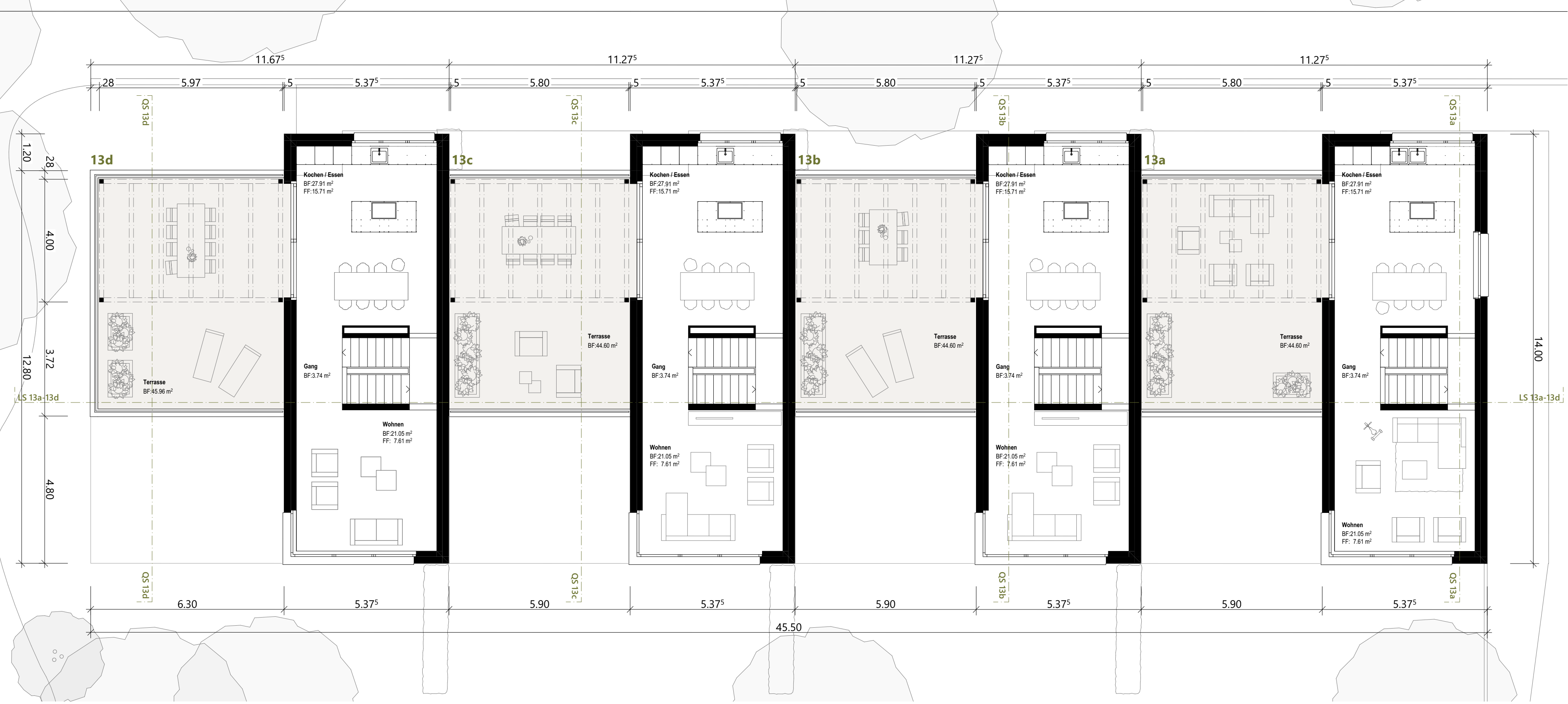
Haus 13a, 13b, 13c und 13d - Obergeschoss
