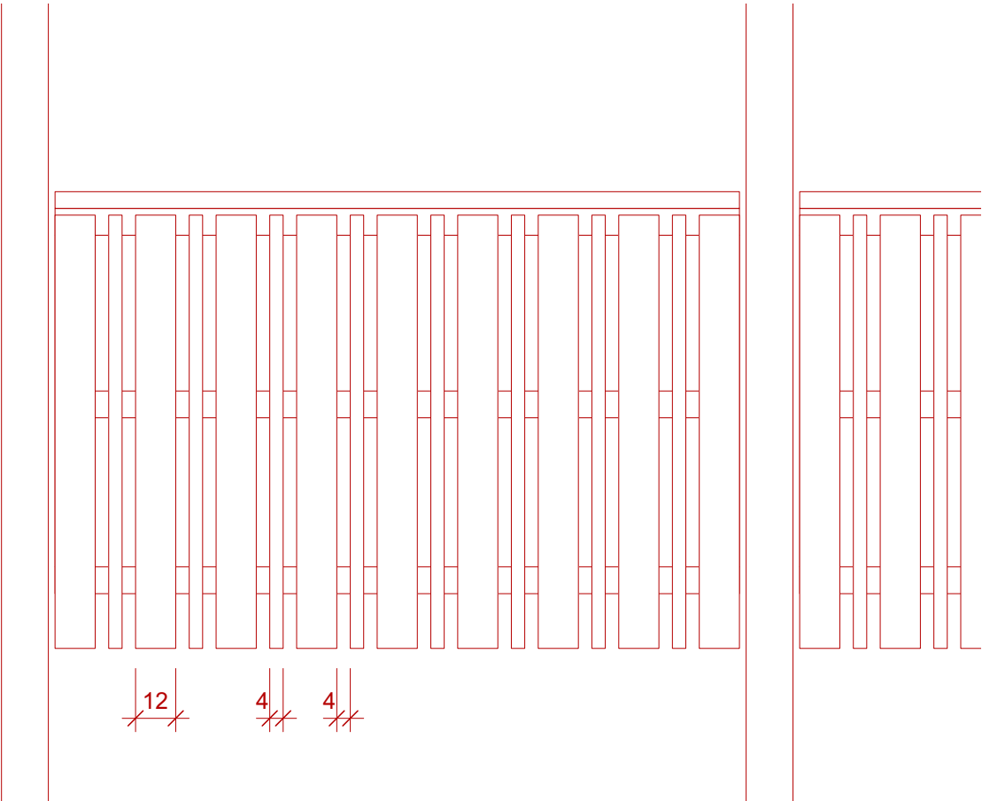
Ansicht
